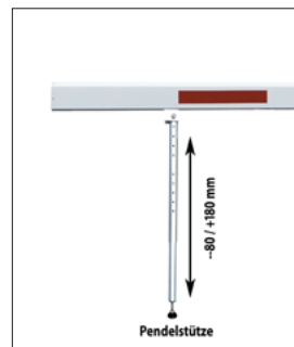
Pendelstütze
