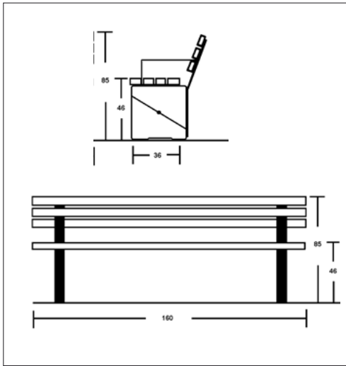
Parkbank „REFLECTION“
