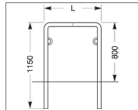
Skizze zum Einbetonieren
