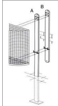
Befestigungsvarianten
